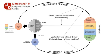
Abbildung 1: Relevanz-Fähigkeits-Vergleich
